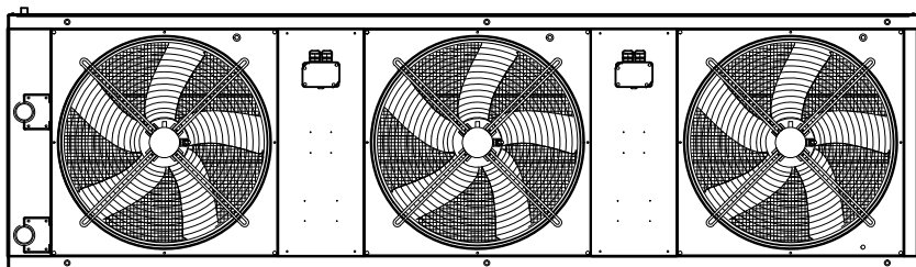
Draufsicht
