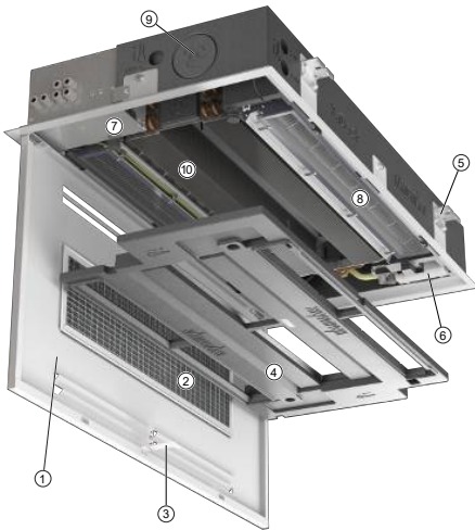
KaDeck en un coup d'œil (exemple soufflage bilatéral, refroidissement humide)
