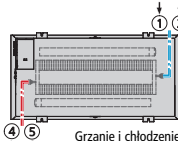
Zawór niezależny od różnicy ciśnienia, większy niż 420 l, 4-przewodowy
