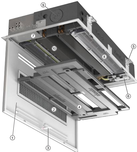
Overzicht KaDeck (voorbeeld tweezijdig uitblazend, vochtige koeling)
